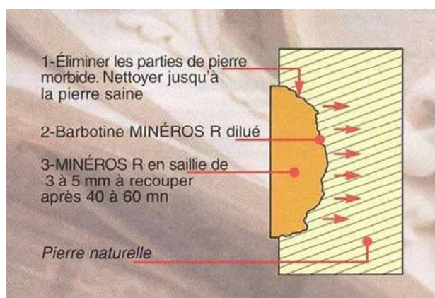
BOUCHON A BASE DE MINEROS R
