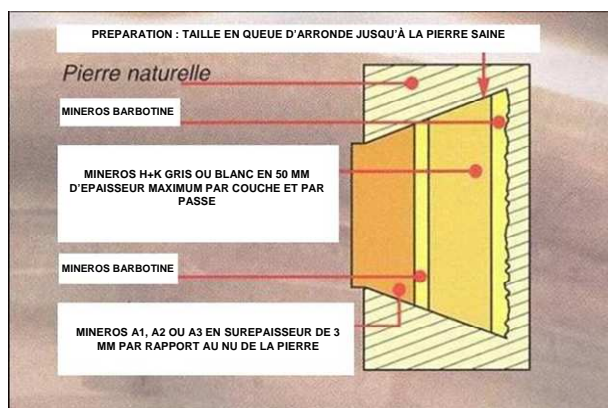
BOUCHON A BASE DE MINEROS H+K & MINEROS A
