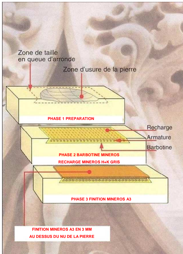
REFECTION DE MARCHES D'ESCALIERS
