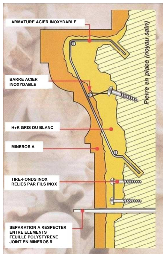
SCHEMA DE CORNICHE OU BANDEAU
